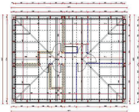
Plancher haut Étage
