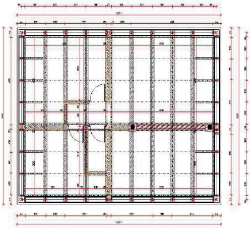
Plancher haut Rez de chaussée
